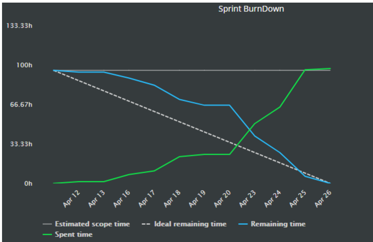
Obrázok 1 Burndown chart
